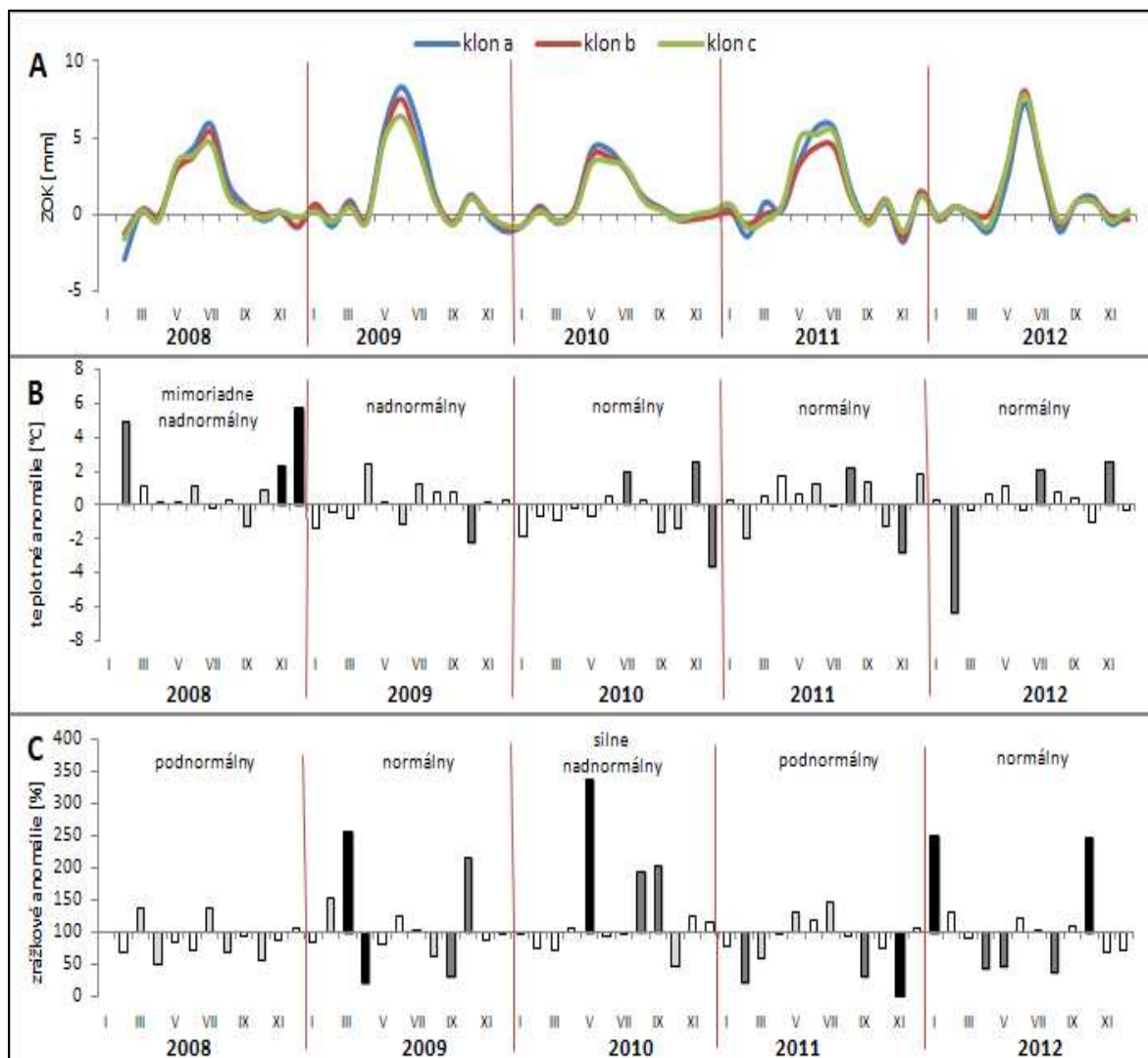
Obr. 3: Rastové krivky mesačných hodnôt zmien obvodu kmeňov ZOK (A). Anomálie teplôt vzduchu AT (B), zrážok P (C) od dlhodobých priemerov, (biela – v rámci normálu, šedá – nad- a podnormálne, tmavo šedá – silne nad a podnormálne, čierna – extrémne pod- a nadnormálne)
