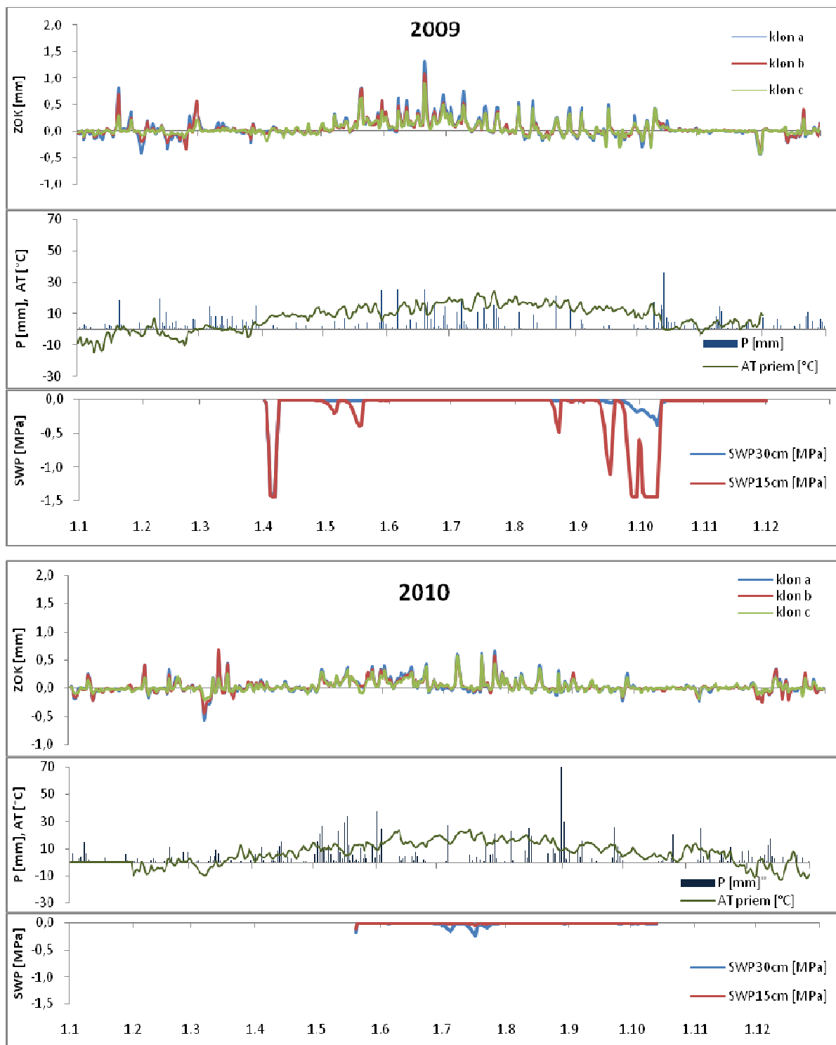
Obr. 4 Denná dynamika zmien obvodu kmeňov (ZOK) a priebeh klimatických (P, AT) a pôdných (SWP) charakteristík v dvoch klimaticky odlišných rokoch 2009 a 2010.
